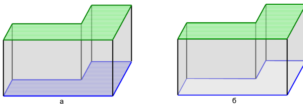
Ү.12-р зураг - LoD1 нь барилга байгууламжийг GM_Solid (а) ба GM_MultiSurface (б) хэлбэрээр дүрсэлнэ.
