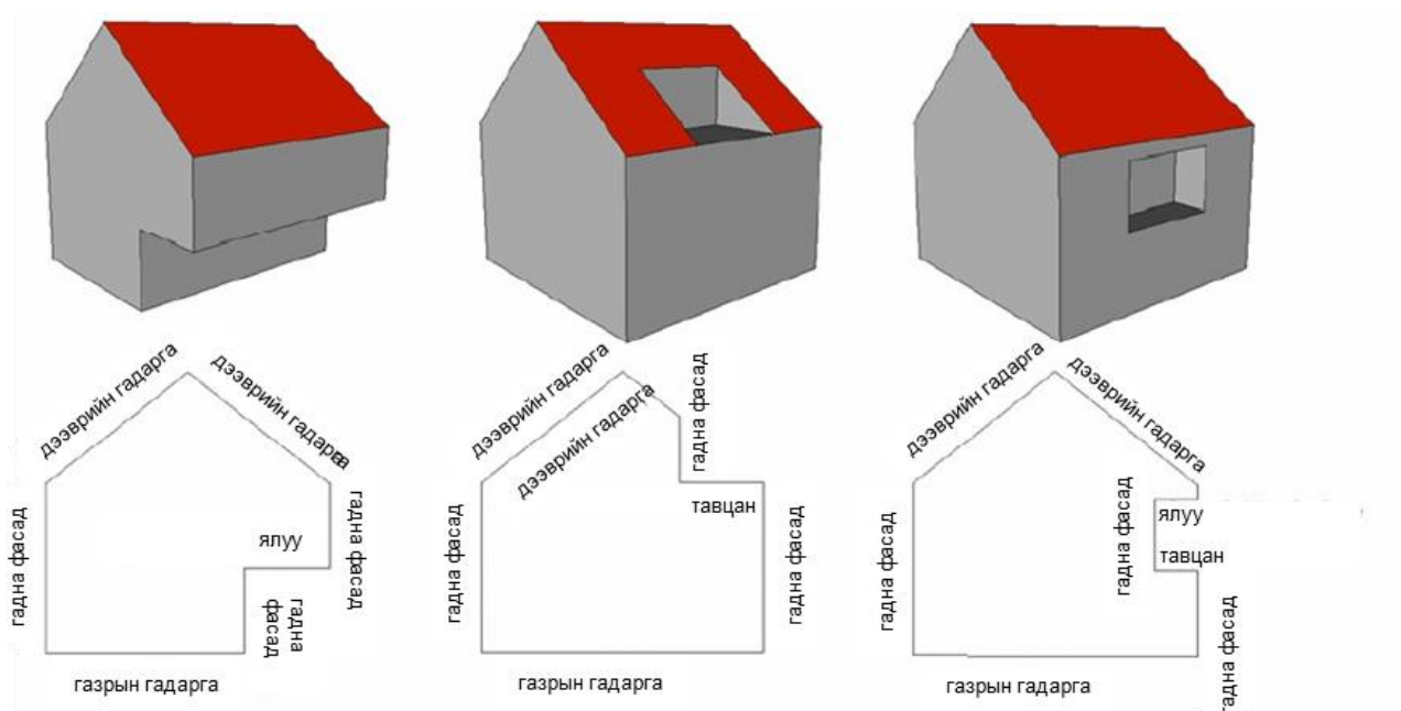
Ф.14-р зураг – Барилга ба барилгын хэсгийн 3 хэмжээст геометр (LoD1-ийн жишээ)
