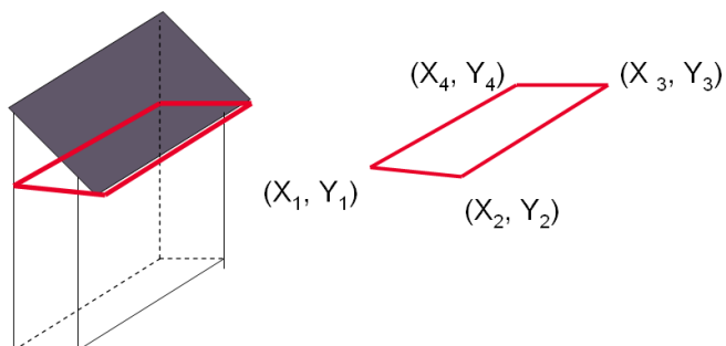
F.1-р зураг – 2 хэмжээст өгөгдлөөр илэрхийлэгдсэн барилга
