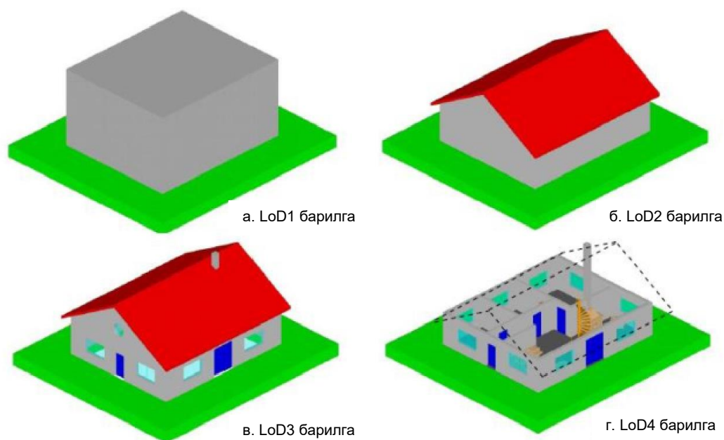
Ү.11-р зураг – Барилгын загварыг нарийвчлан үзүүлэх 4 түвшин (CityGML)
