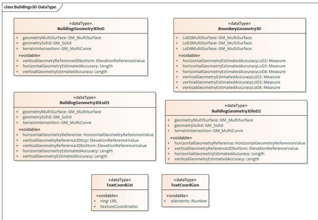
С.7-р зураг - UML диаграмм: 3 хэмжээст барилга - Өгөгдөл төрлүүдийн тойм
